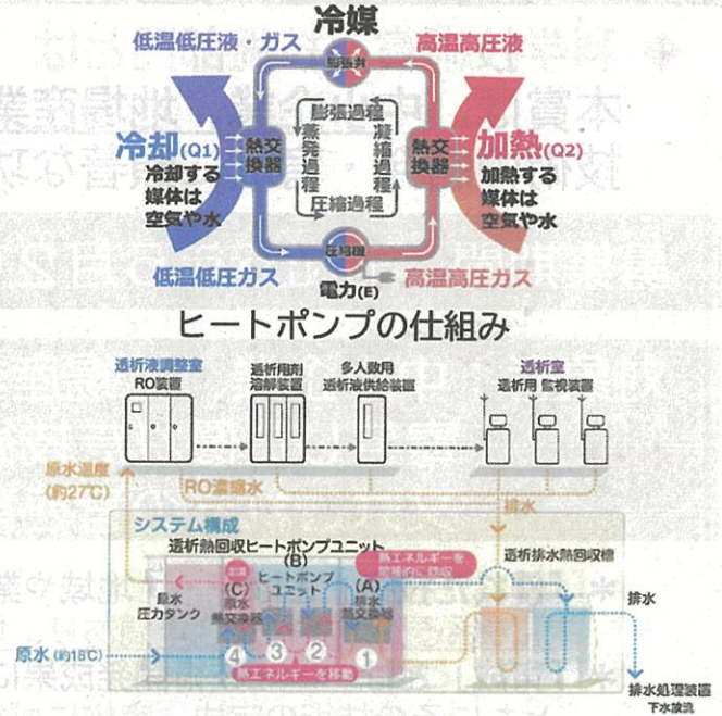
透析熱回収ヒートポンプシステム
